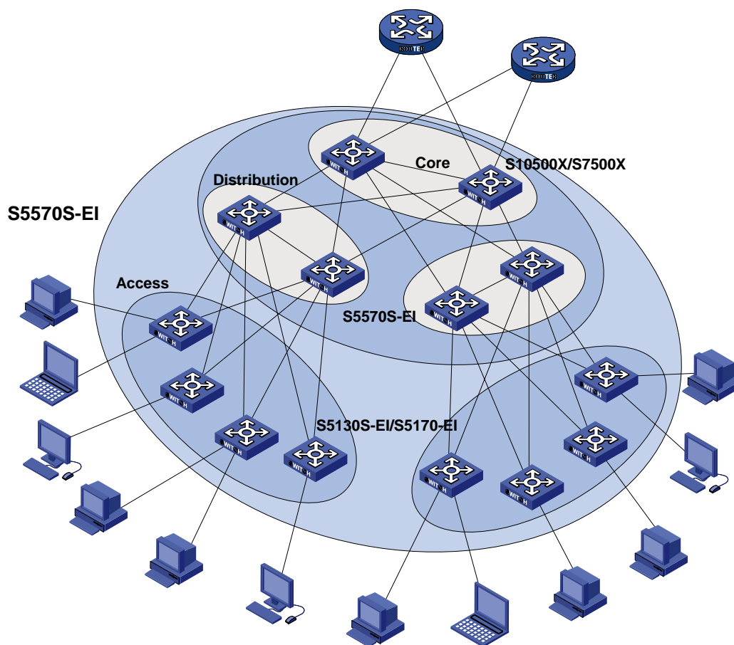
S5570S-EI汇聚层组网应用
