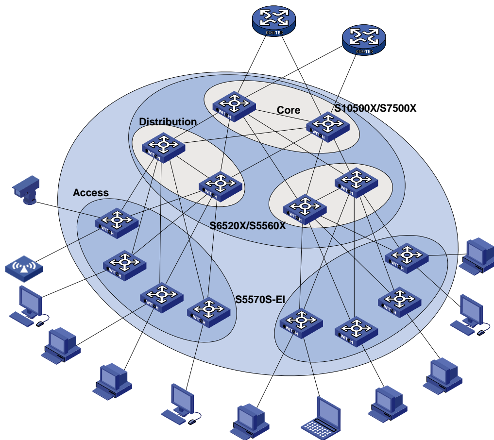
S5570S-EI接入层组网应用
