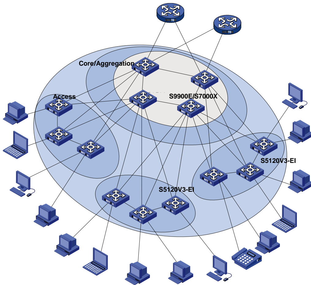
S5120V3-EI接入层组网应用
