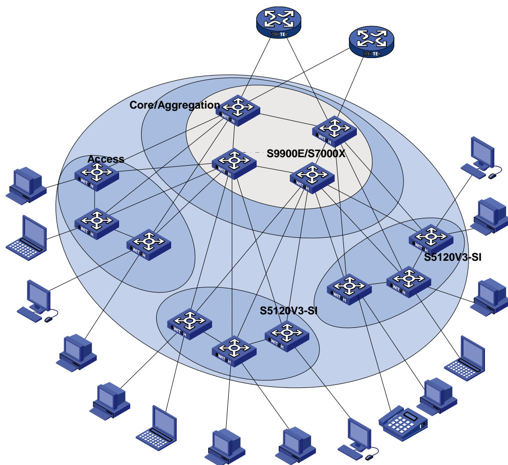
S5120V3-SI接入层组网应用
