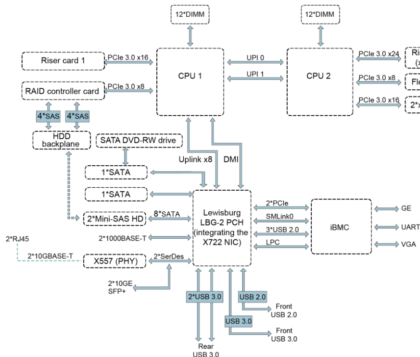
图4-1 1288H V5 逻辑结构
