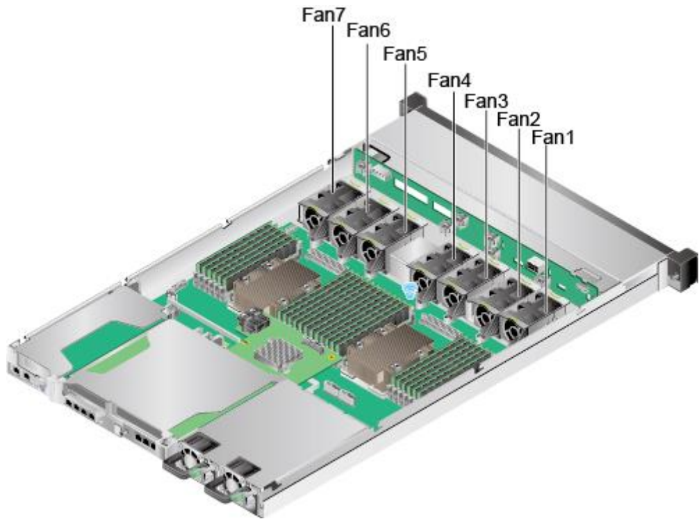
图5-39 风扇位置
