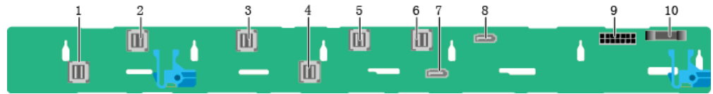
图5-43 10x2.5 英寸硬盘背板 1 (BOM: 03024KYL)
