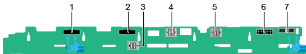
图5-44 10x2.5 英寸硬盘背板 2 (BOM: 03025CYT、03029VWF)
