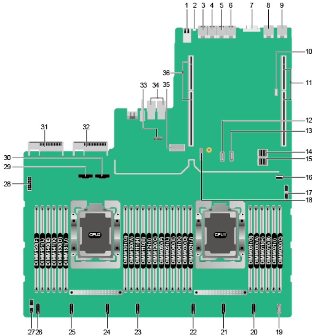
图5-40 1288H V5 主板（BOM：03024AFS、03029JRW、03024CXR、03029JRV）
