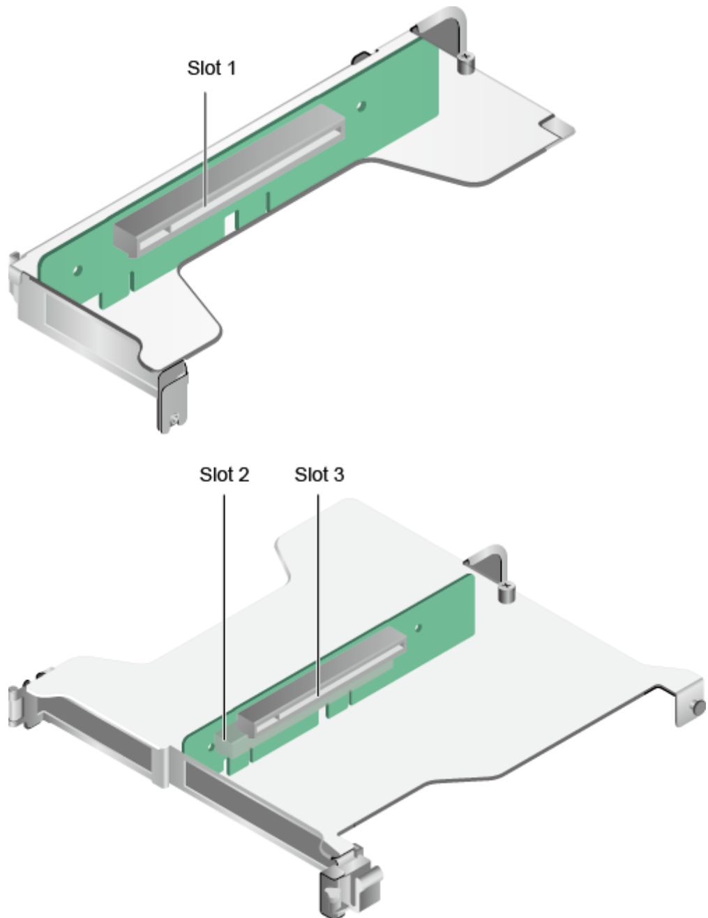
图5-37 PCIe Riser 模组
