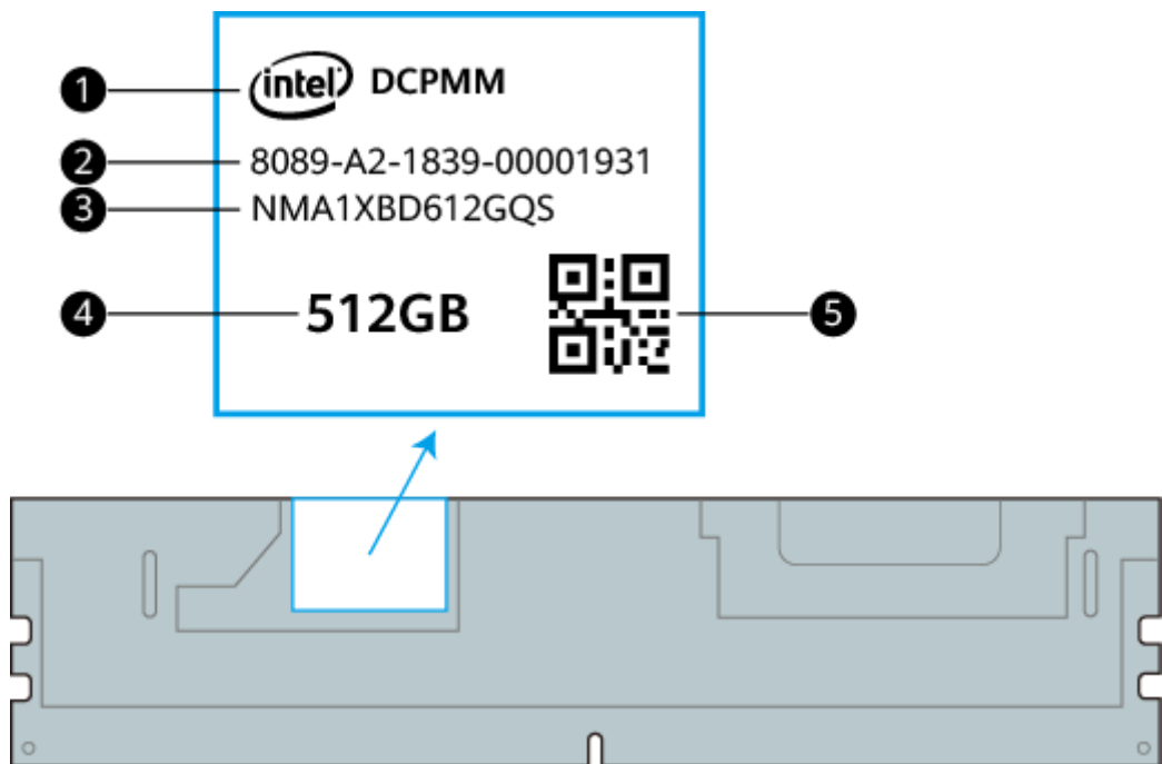
图5-18 内存标识
