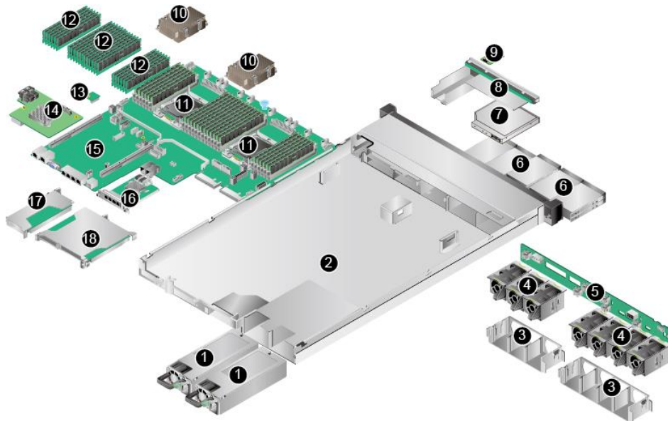
图3-1 1288H V5 物理结构（示例：8x2.5 英寸硬盘配置）
