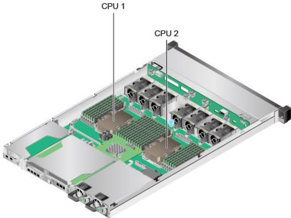
图5-13 处理器位置
