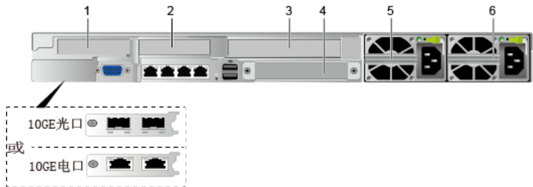
图5-10 后面板外观
