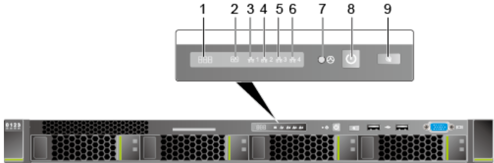
图5-4 前面板指示灯和按钮
