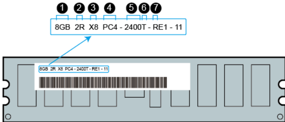
图5-14 内存标识
