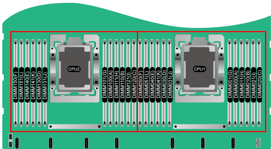
图5-15 内存插槽位置
