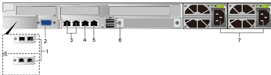
图5-12 后面板接口
