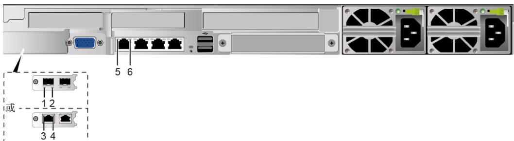
图5-29 板载网卡指示灯
