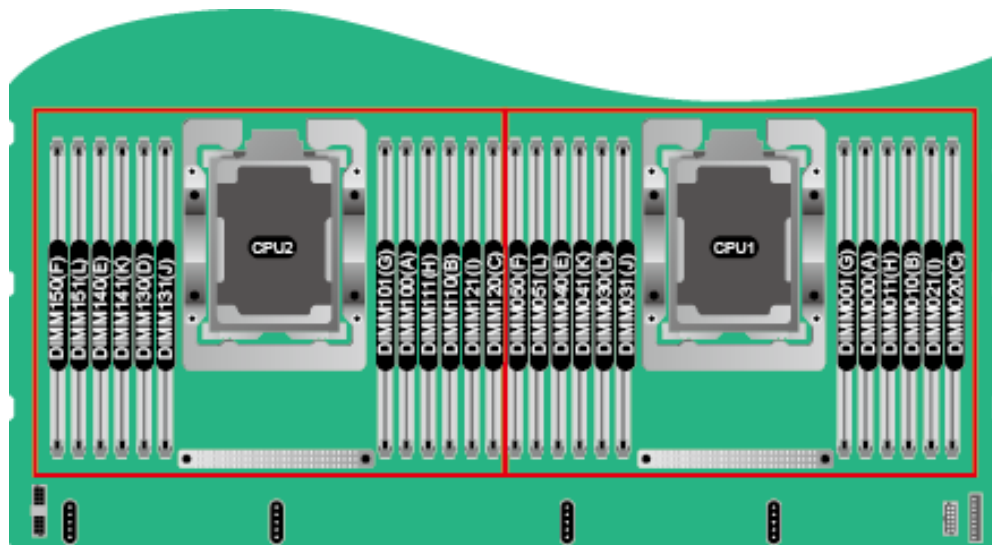
图5-19 内存插槽位置
