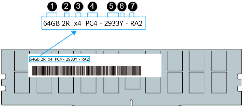
图5-14 内存标识
