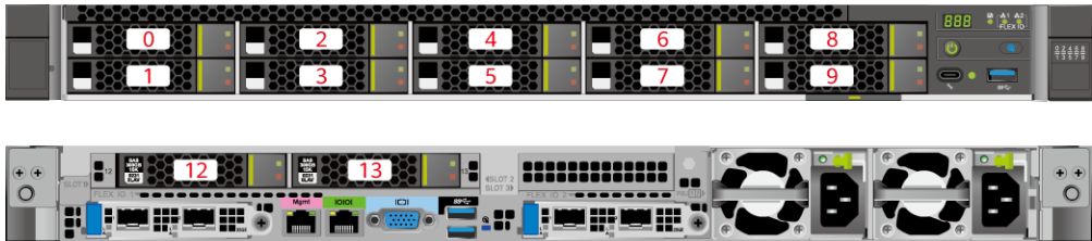
图5-23 硬盘编号
