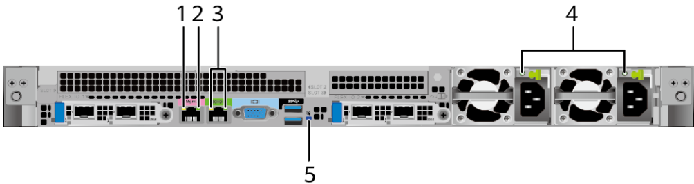
图5-11 后面板指示灯
