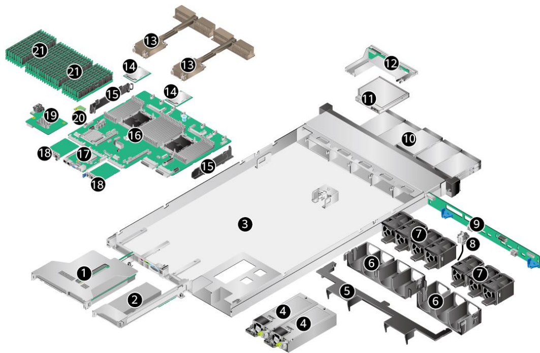
图3-1 物理结构（示例：8x2.5 英寸硬盘配置）
