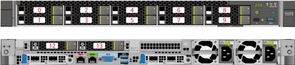
图5-28 硬盘编号
