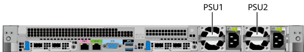
图5-35 电源模块位置
