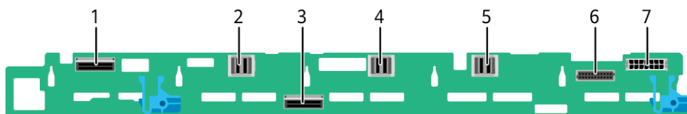
图5-40 10x2.5 英寸硬盘直通配置背板
