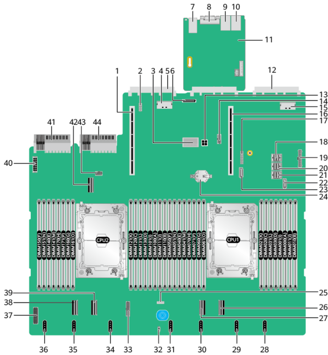
图5-37 1288H V6 主板
