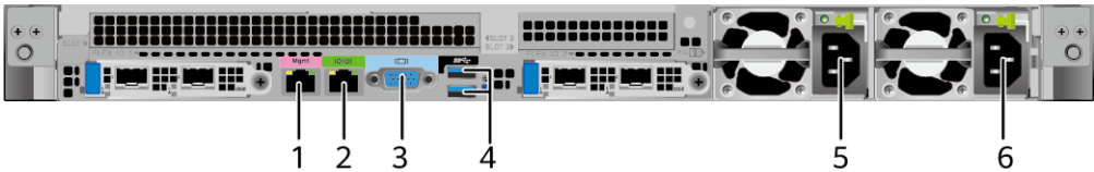
图5-12 后面板接口
