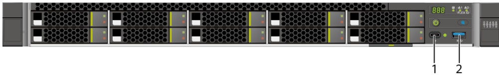
图5-9 前面板接口
