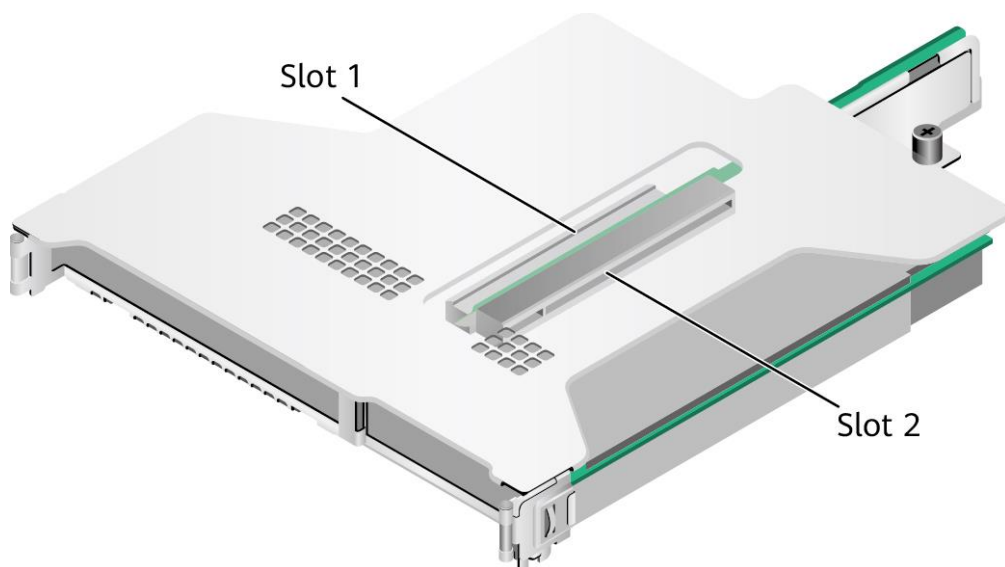
图5-33 PCIe Riser 模组
