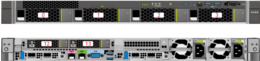
图5-19 硬盘编号
