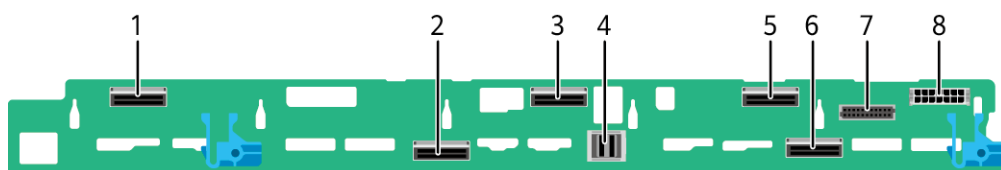
图5-41 10x2.5 英寸硬盘 NVMe 配置背板
