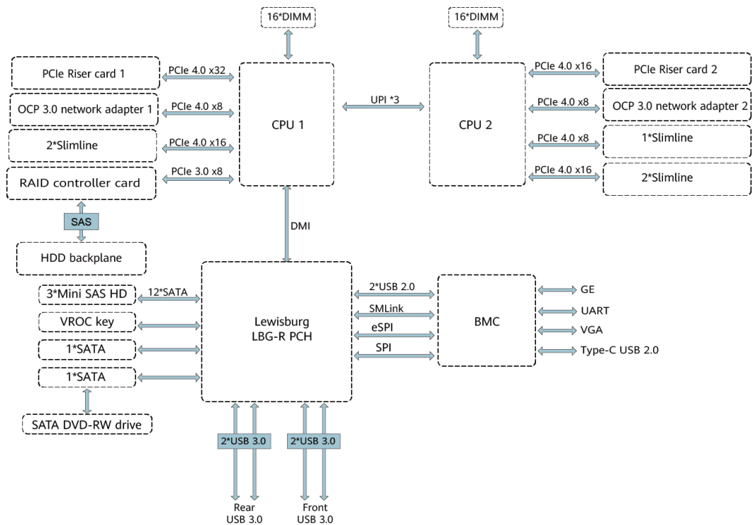
图4-1 逻辑结构
