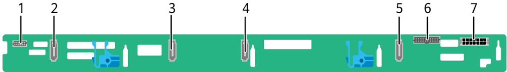
图5-38 4x3.5 英寸硬盘直通配置背板
