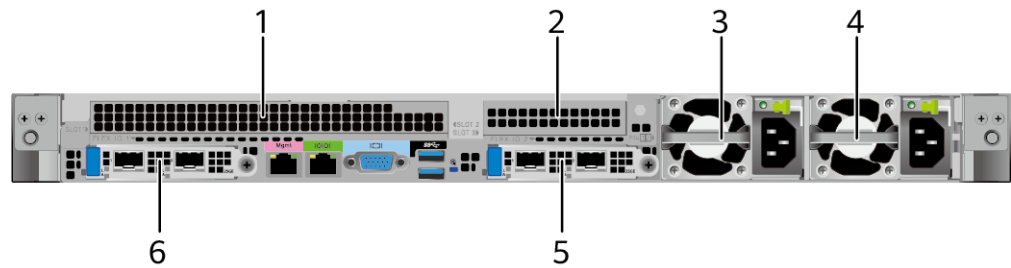
图5-10 后面板外观
