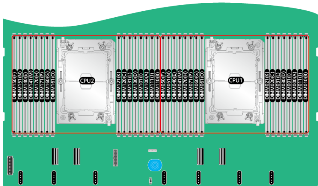
图5-15 内存插槽位置
