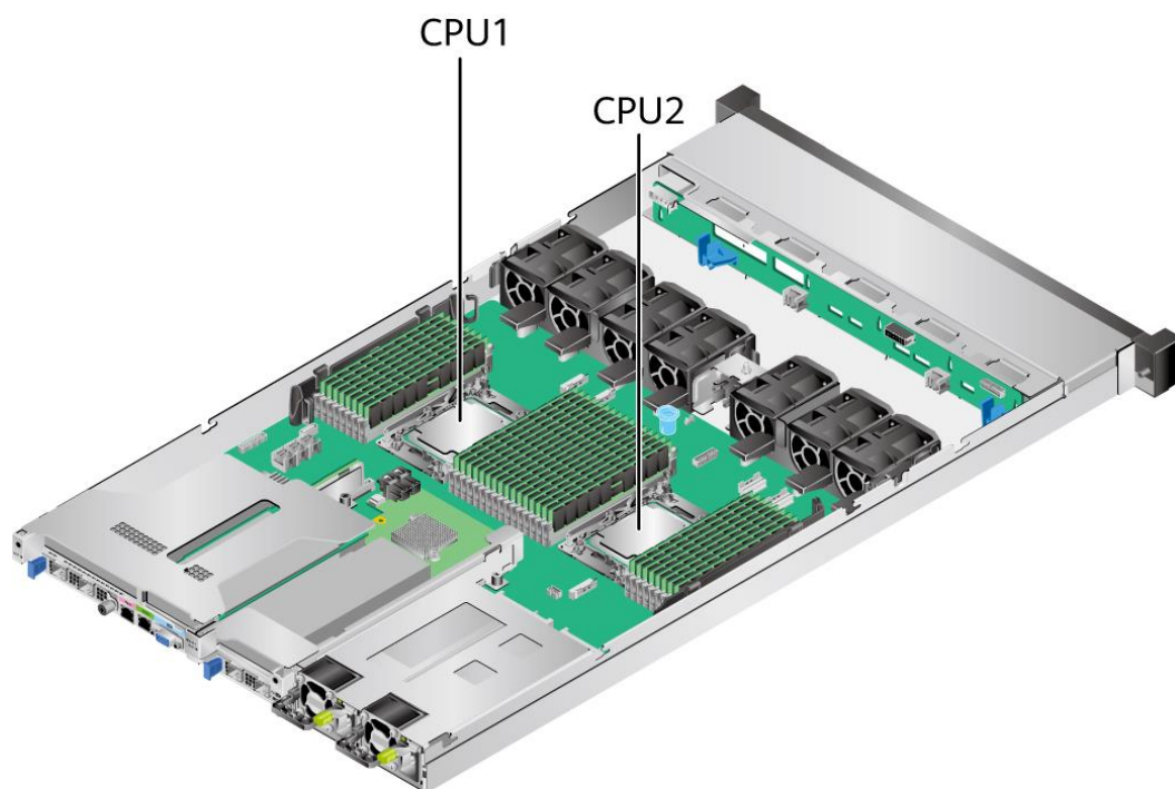
图5-13 处理器位置
