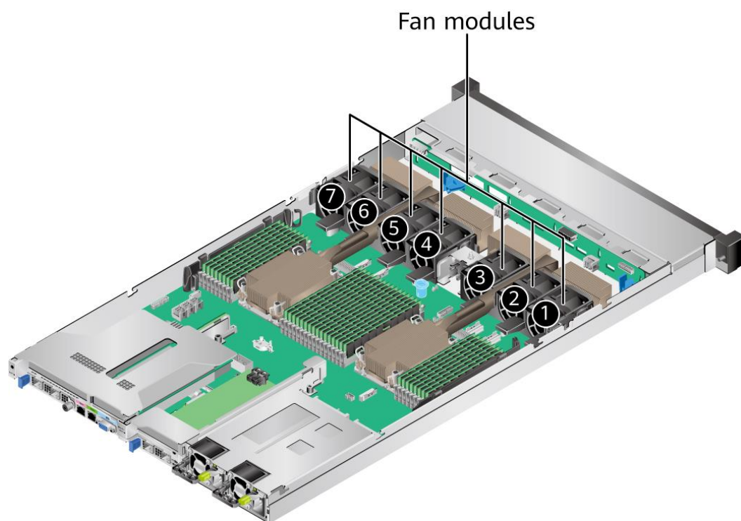
图5-36 风扇模块的位置
