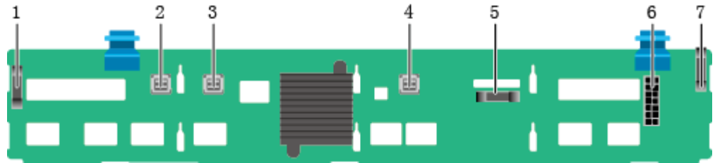
图5-64 12x3.5 英寸硬盘 EXP 配置背板 (BOM: 03024DDH、03024MSG、03029JSA)
