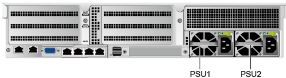
图5-60 电源位置
