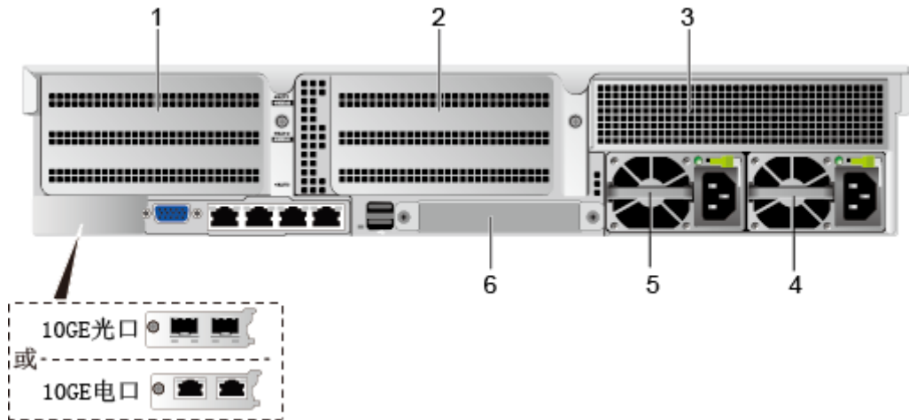
图5-16 后面板外观
