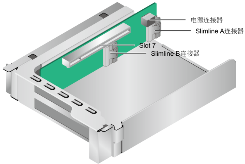
图5-58 PCIe Riser 模组 6
