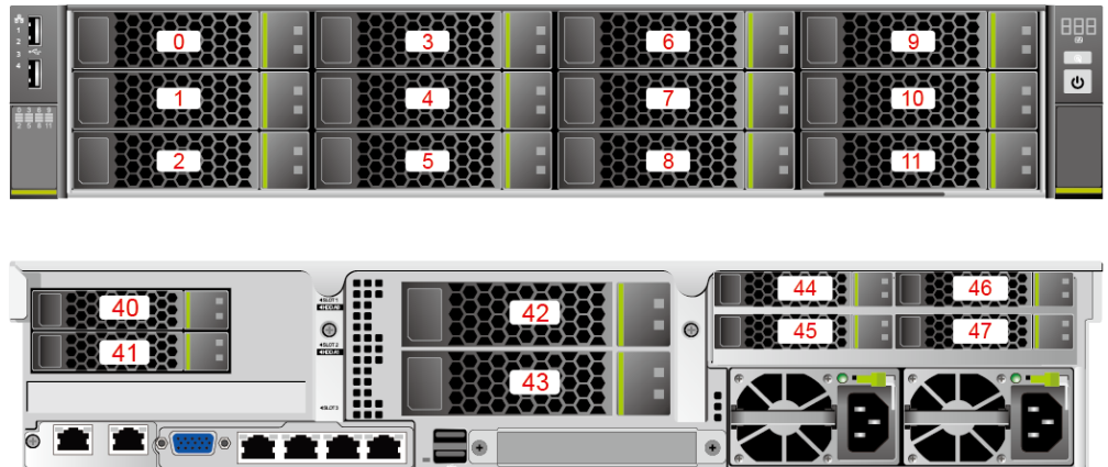
图5-33 硬盘编号
