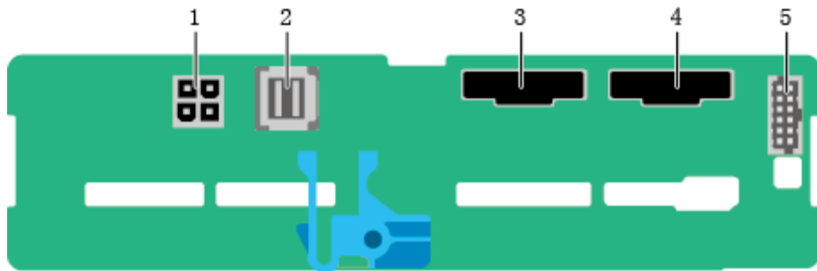
图5-73 4x2.5 英寸硬盘背板 (BOM: 03024BPV、03029TDR)
