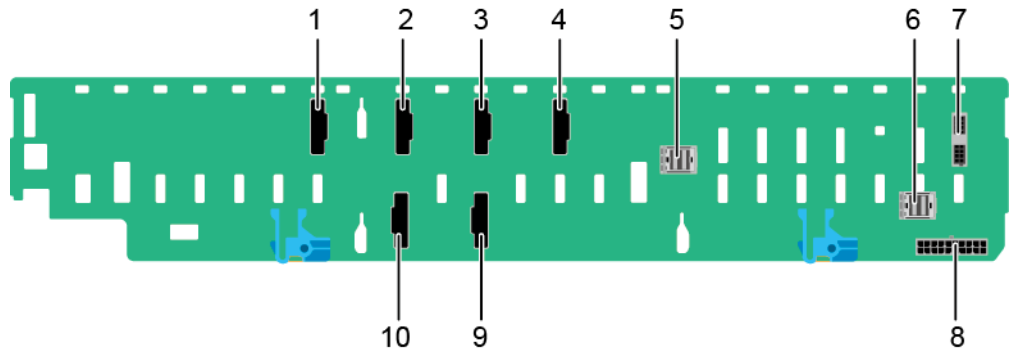
图5-66 20x2.5 英寸硬盘配置 (8xSAS/SATA+12xNVMe) 背板 (BOM: 03025EUL、03029TDE)
