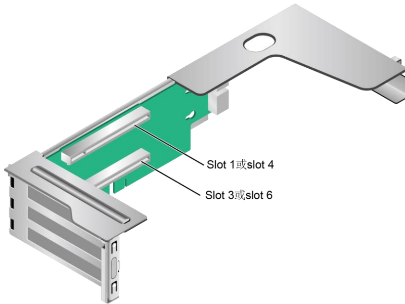
图5-56 PCIe Riser 模组 4
