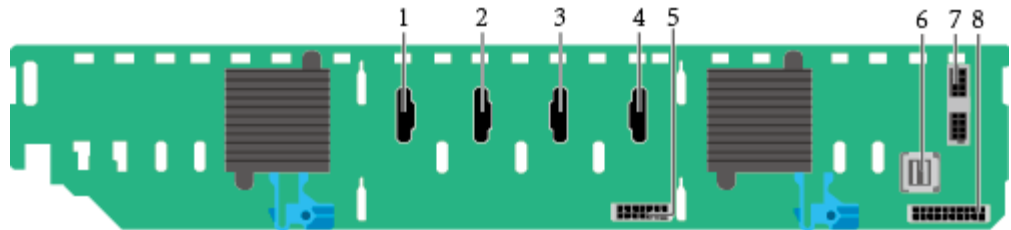
图5-68 24x2.5 英寸硬盘 NVMe 配置背板 (BOM: 03023WAD)
