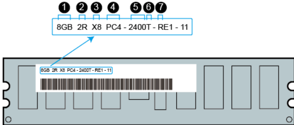
图5-20 内存标识
