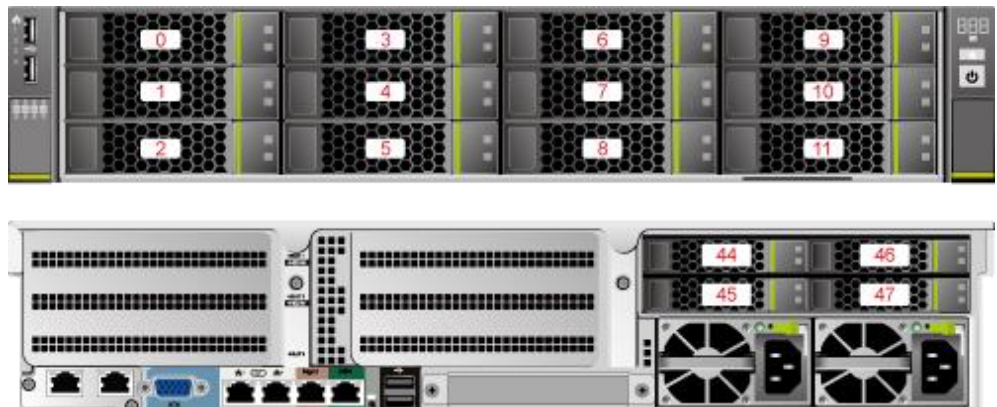
图5-35 硬盘编号
