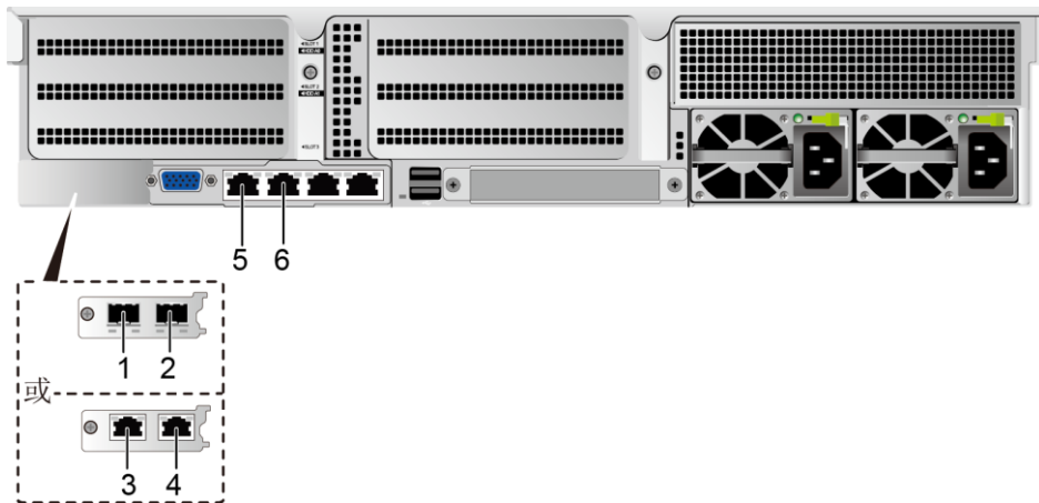
图5-45 板载网口
