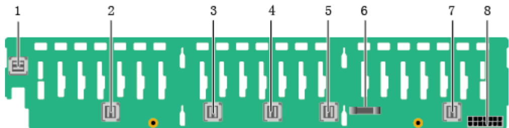
图5-67 24x2.5 英寸硬盘直通配置背板 (BOM: 03022JWW、03029WFE)
