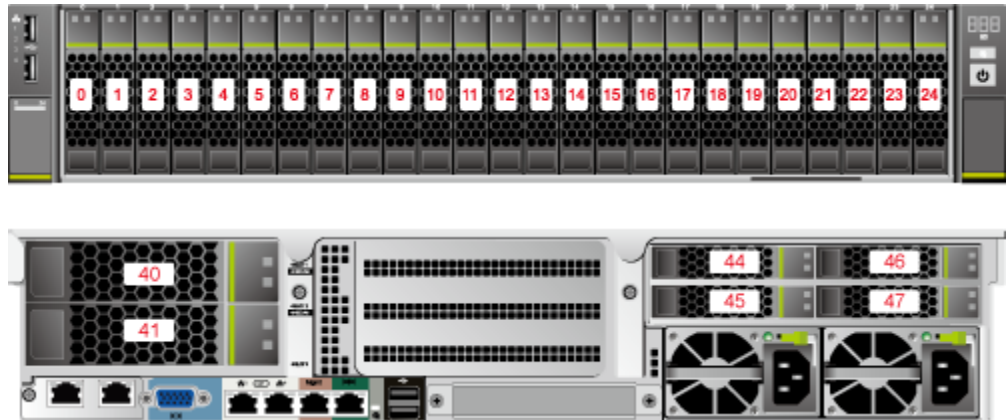
图5-41 硬盘编号
