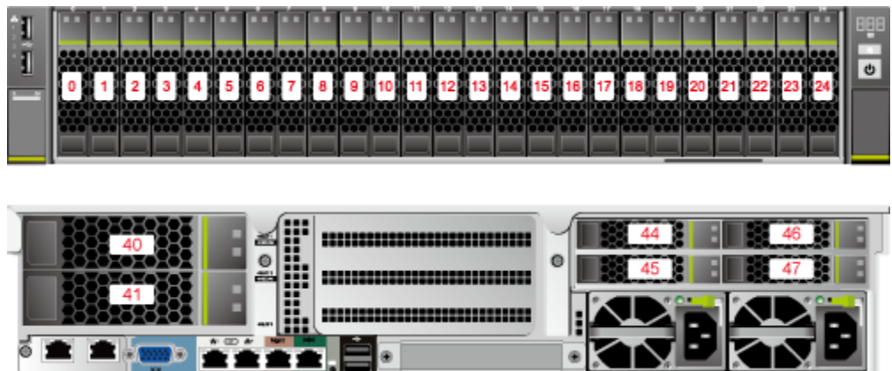
图5-40 硬盘编号
