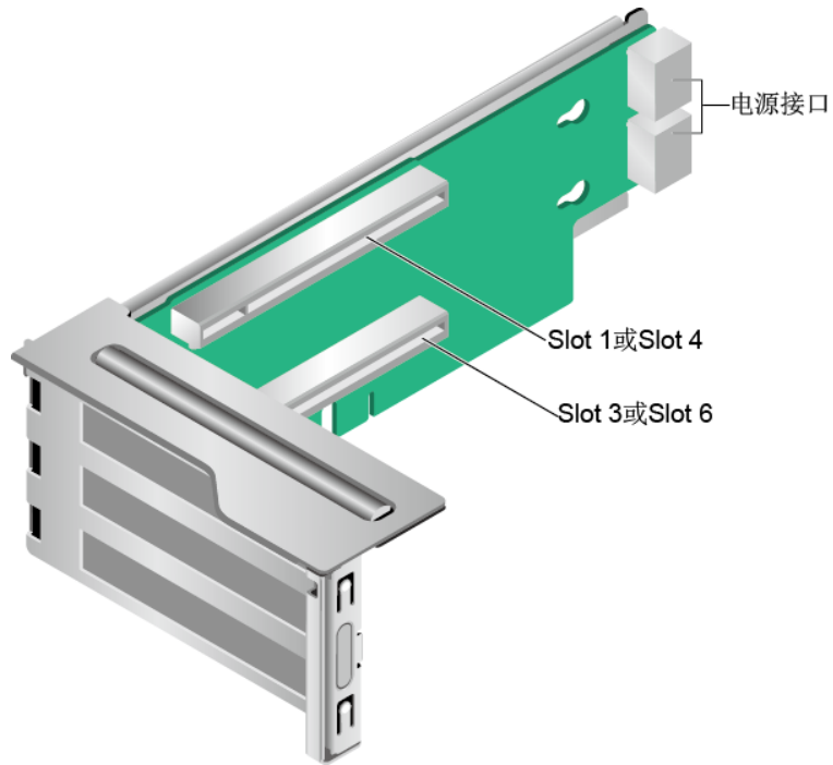
图5-54 PCIe Riser 模组 1
