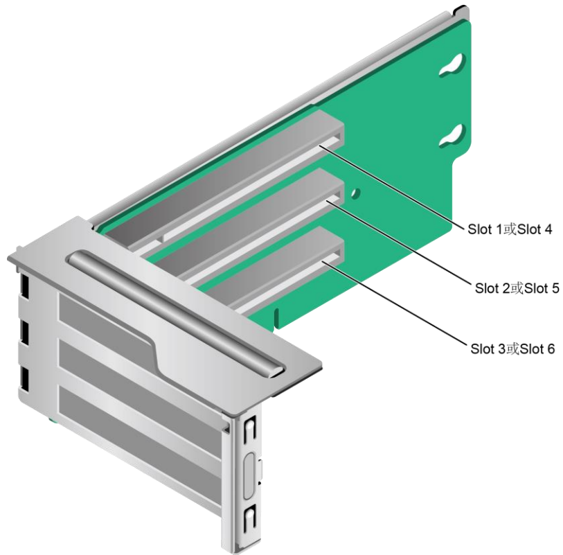
图5-55 PCIe Riser 模组 2
