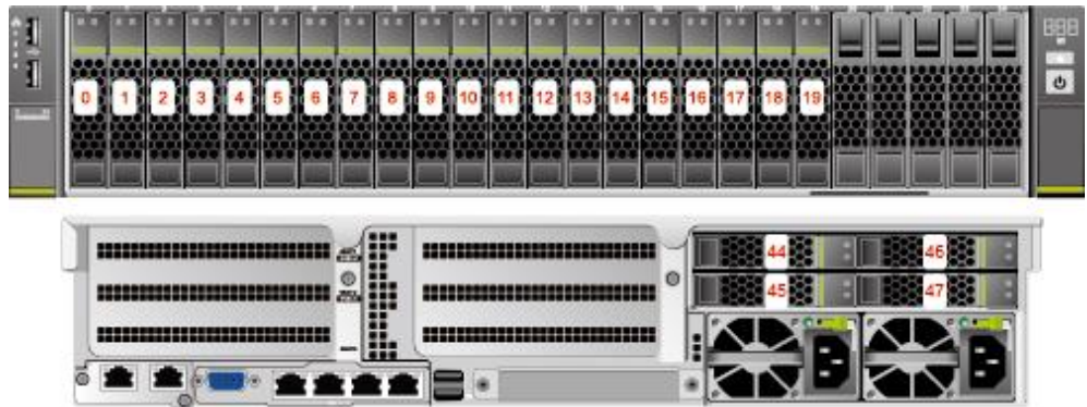
图5-38 硬盘编号
