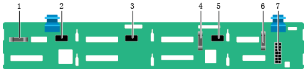
图5-65 12x3.5 英寸硬盘直通配置背板 (BOM: 03024JMV、03029TDH)
