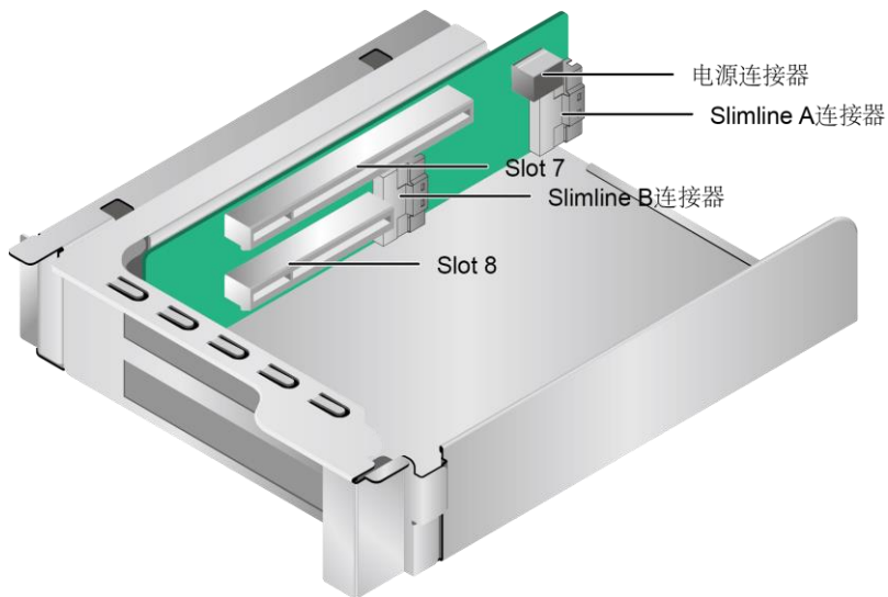
图5-57 PCIe Riser 模组 5
