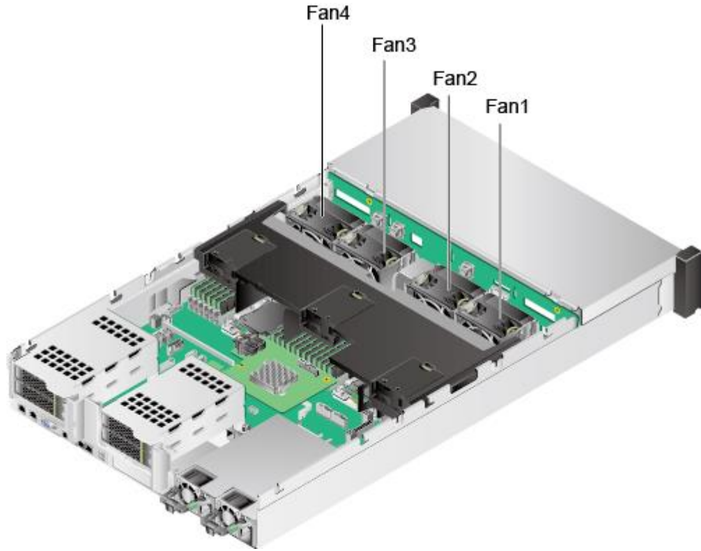
图5-61 风扇位置
