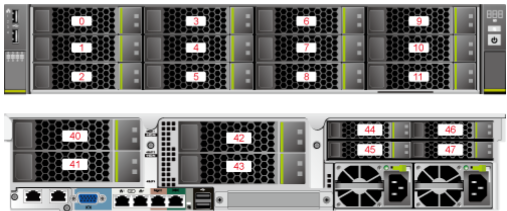
图5-34 硬盘编号
