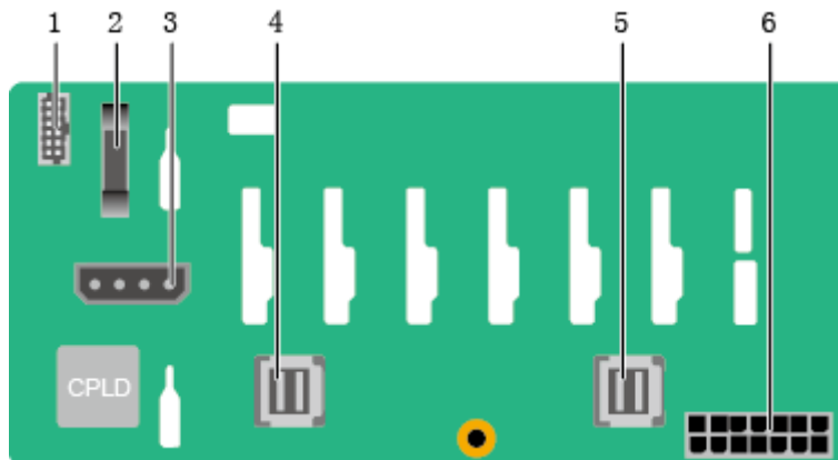
图5-63 8x2.5 英寸硬盘配置背板 (BOM: 03022HXW、03029JRY)
