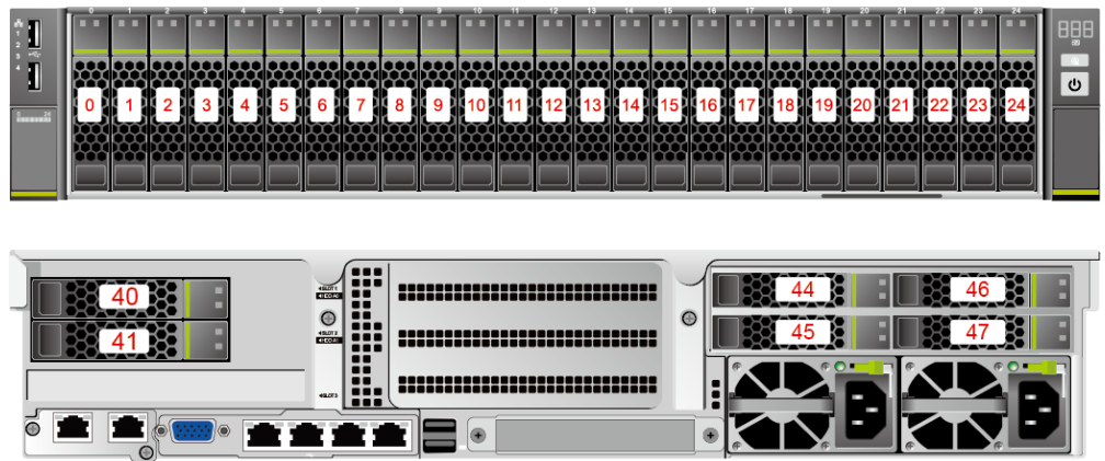
图5-42 硬盘编号
