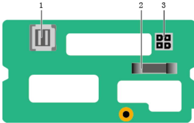
图5-72 2x3.5 英寸硬盘背板 (BOM: 03022HYE)
