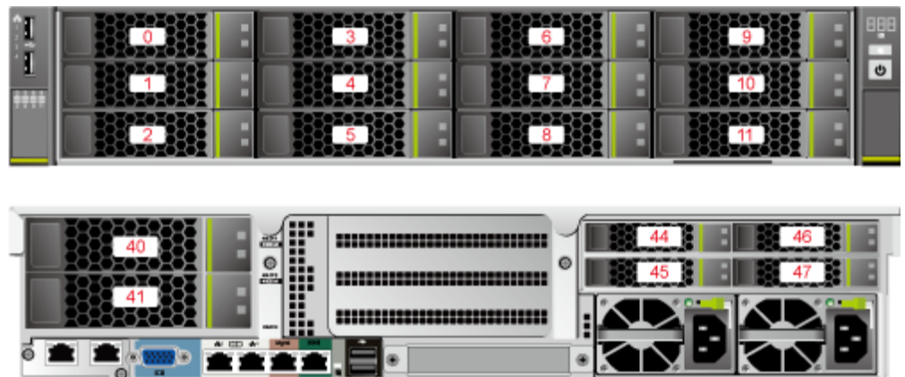
图5-37 硬盘编号
