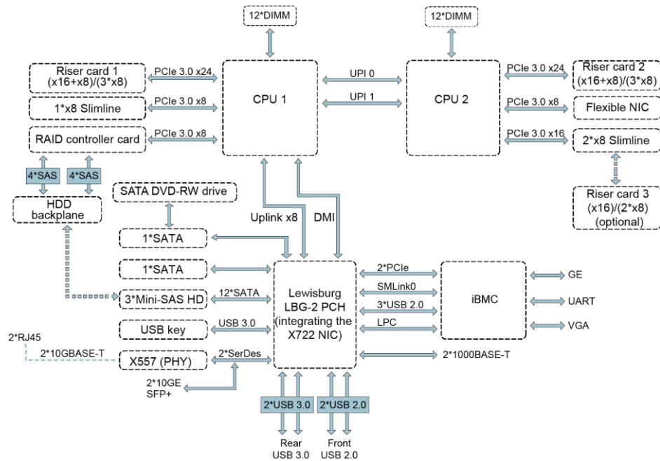
图4-1 2288H V5 逻辑结构
