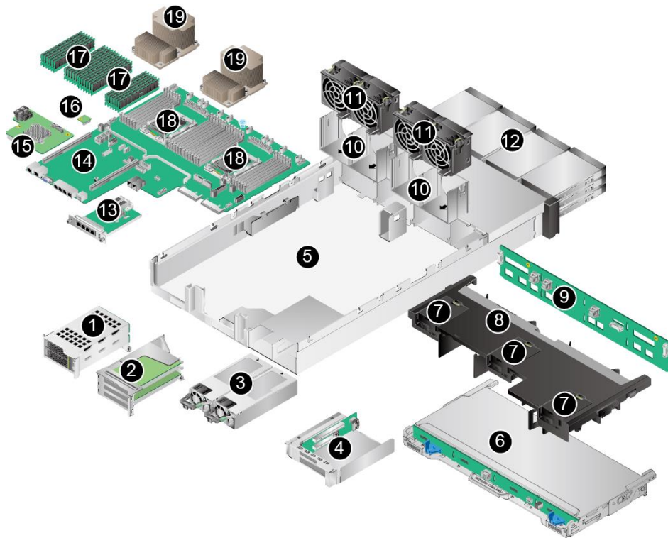
图3-1 2288H V5 物理结构（示例：12x3.5 英寸硬盘配置）
