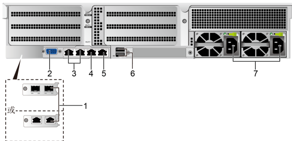
图5-18 后面板接口
