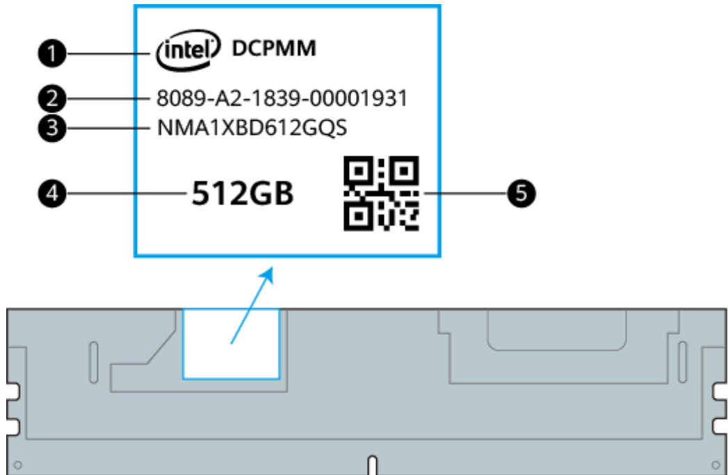
图5-24 内存标识
