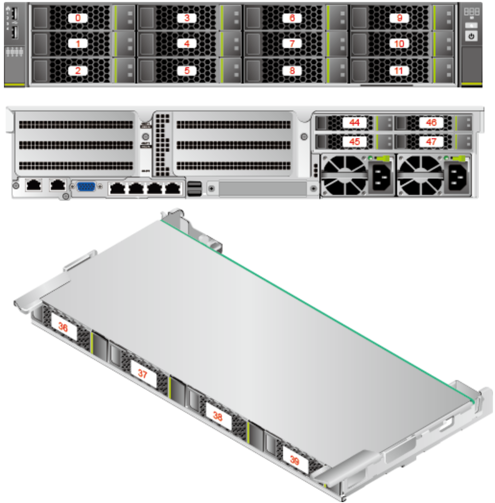
图5-36 硬盘编号
