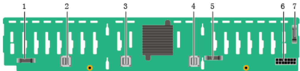
图5-69 25x2.5 英寸硬盘配置背板 (BOM: 03022HYB、03024MSH、03029TDQ)
