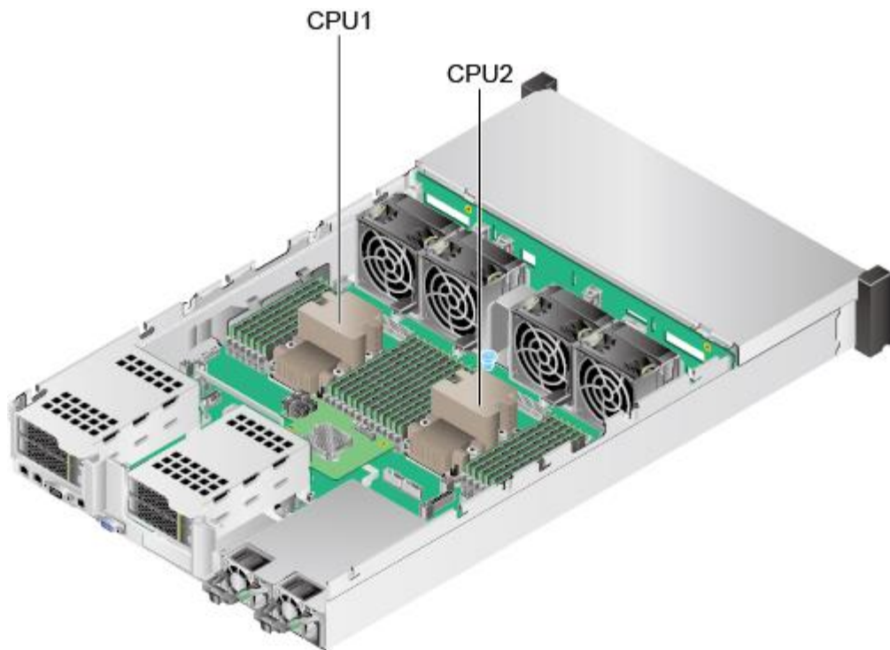
图5-19 处理器位置
