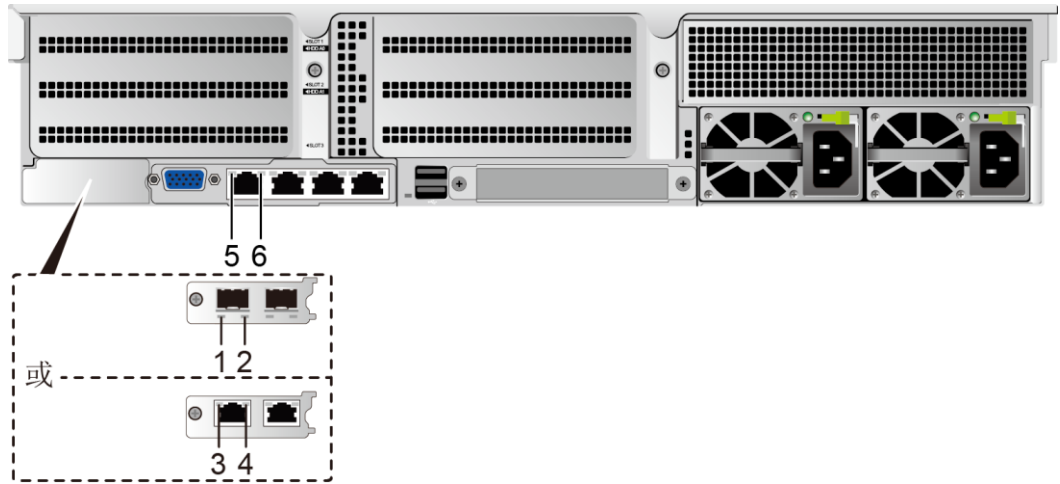
图5-46 板载网卡指示灯
