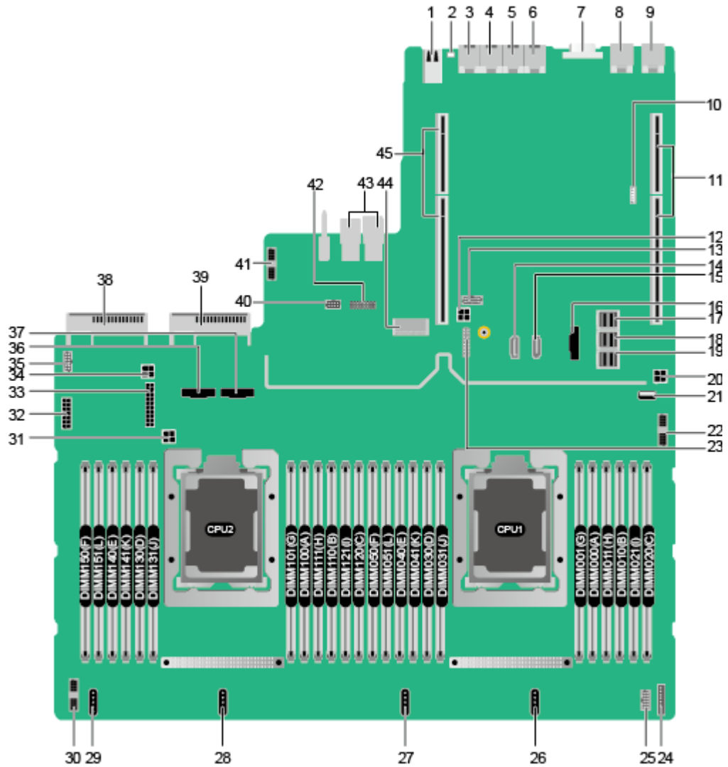
图5-62 2288H V5 主板（BOM：03024AFQ、03026NEA、03024CXS、03029JRP）
