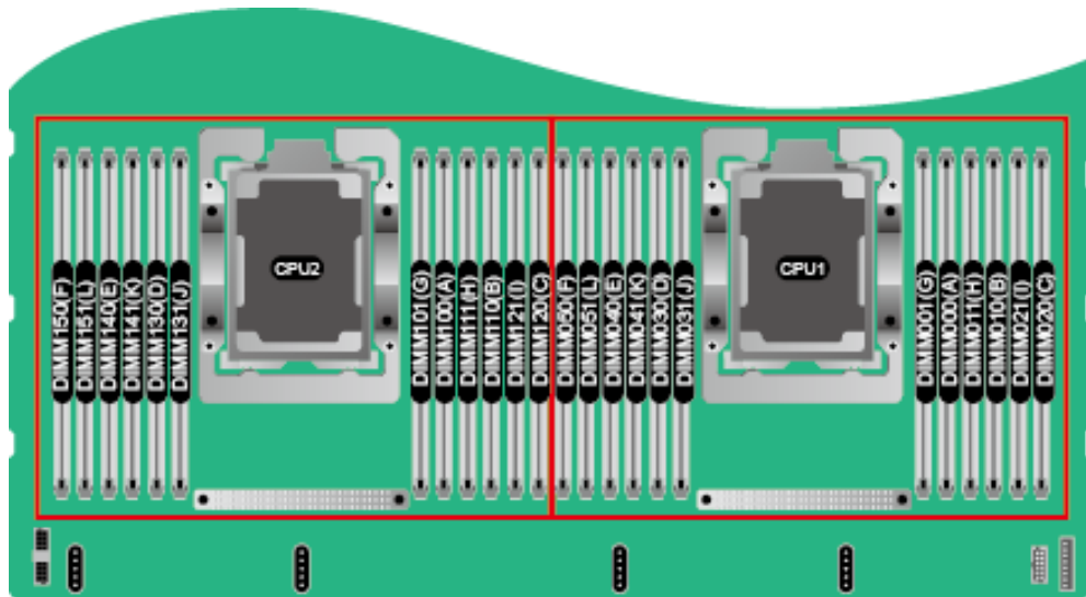
图5-25 内存插槽位置
