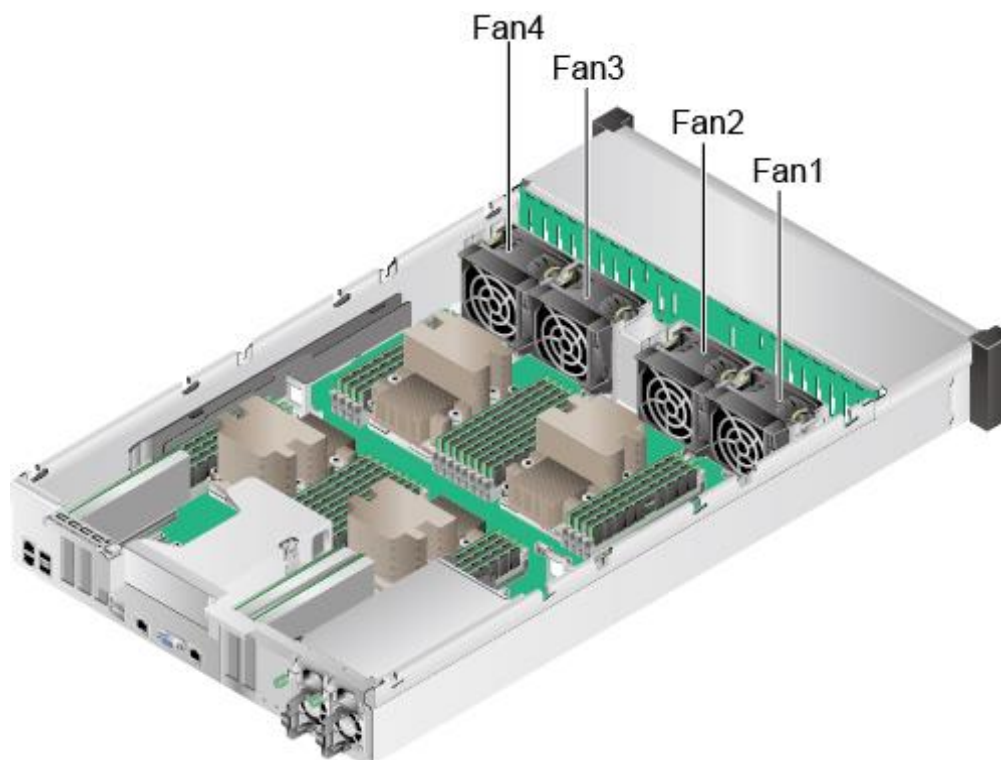
图5-27 风扇位置
