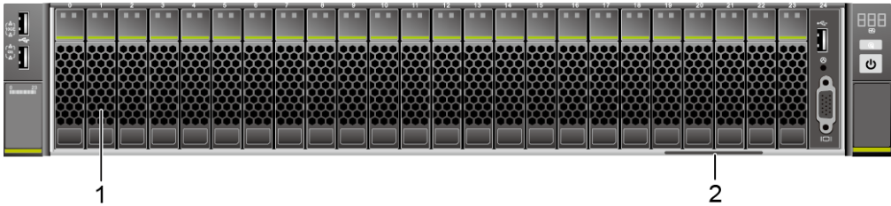
图5-2 前面板外观
