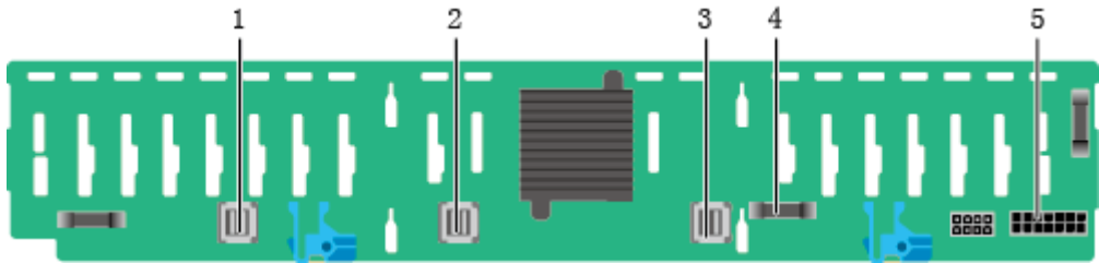
图5-33 25x2.5 英寸硬盘背板 (25xSAS/SATA)
