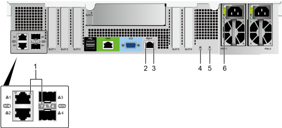
图5-11 后面板指示灯
