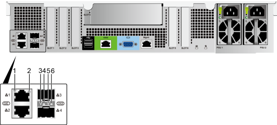
图5-24 板载网卡指示灯
