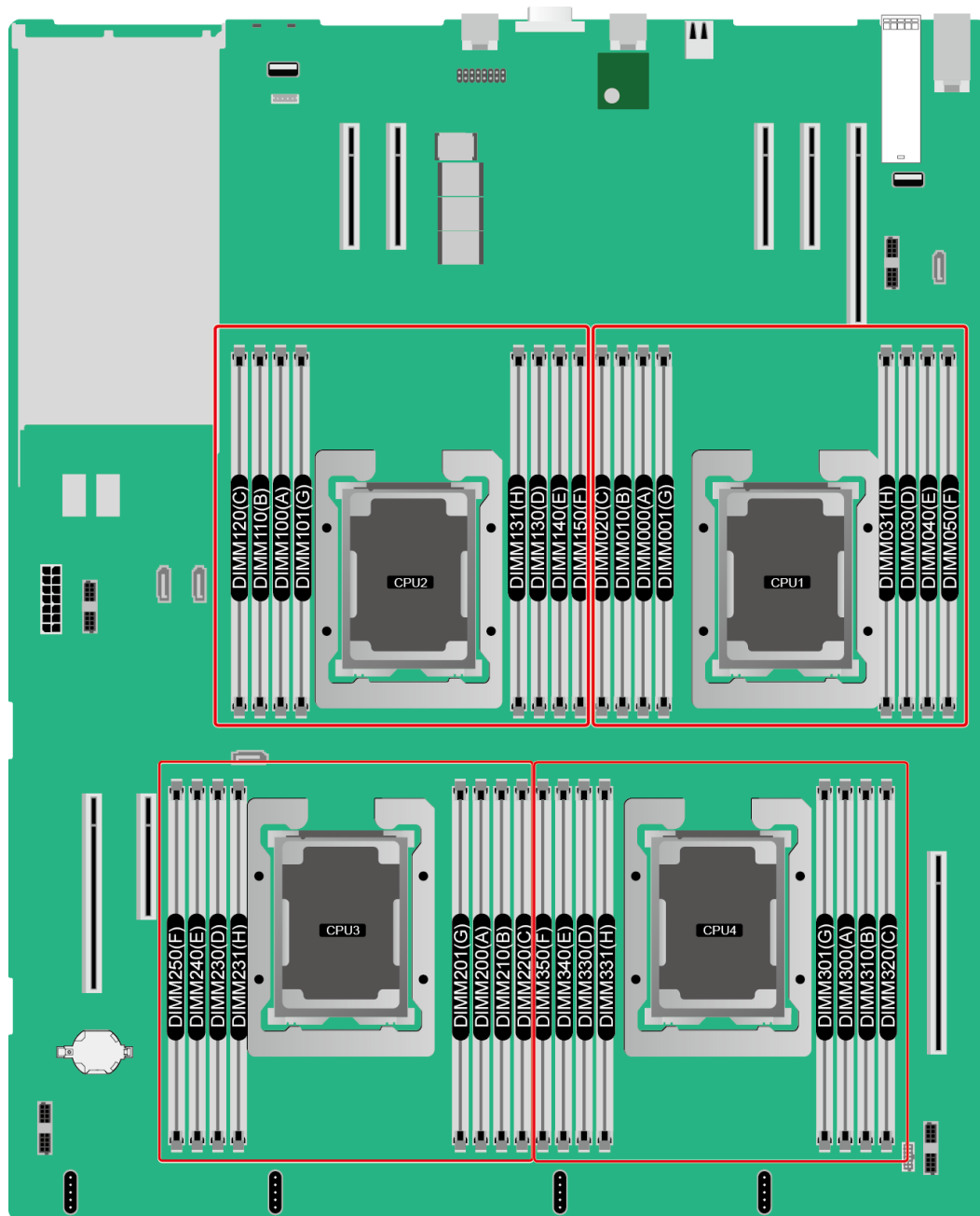
图5-15 内存插槽位置
