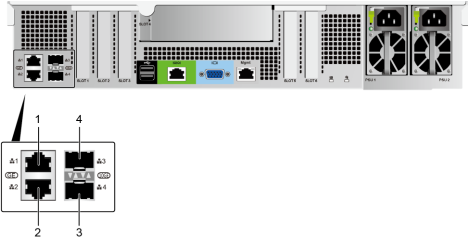
图5-23 板载网口
