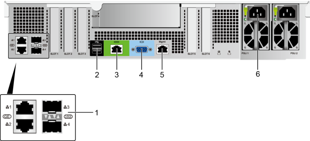
图5-12 后面板接口
