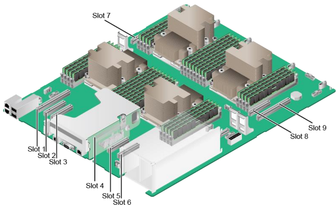
图5-25 PCIe 插槽
