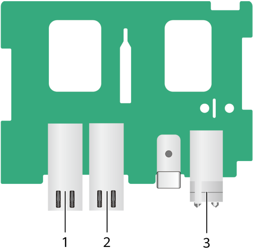
图5-34 2488 V5 电源背板
