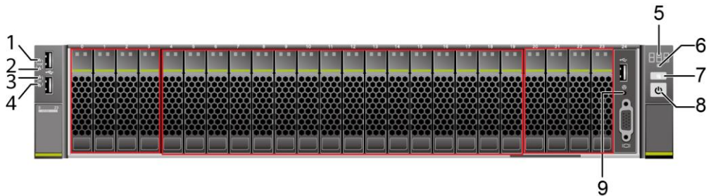
图5-5 前面板指示灯和按钮
