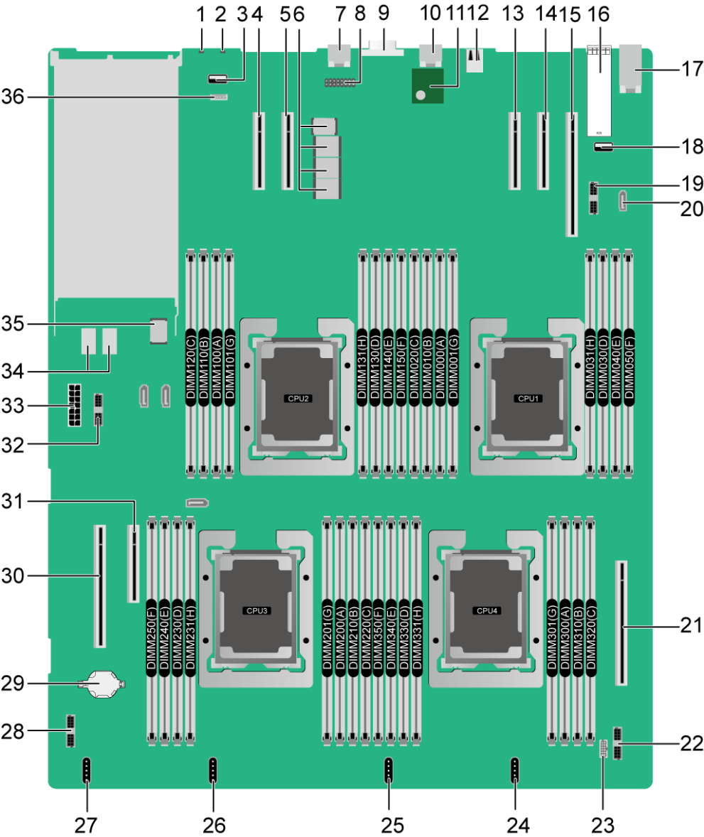
图5-30 2488 V5 主板
