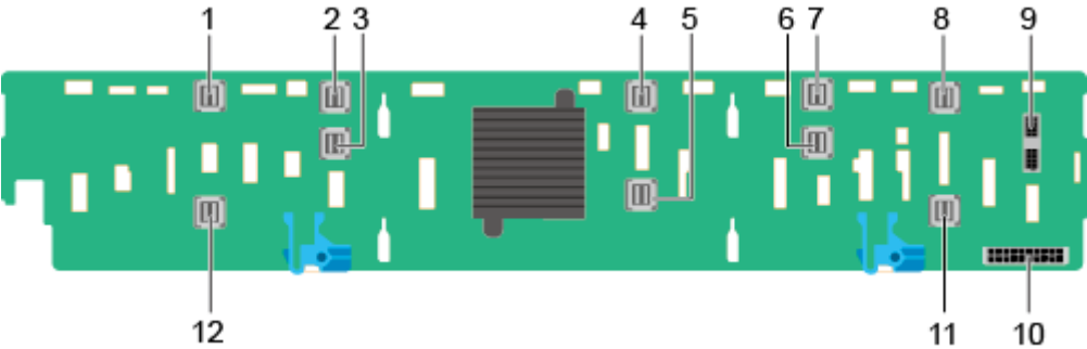
图5-32 24x2.5 英寸硬盘背板（16xSAS/SATA+8xNVMe）
