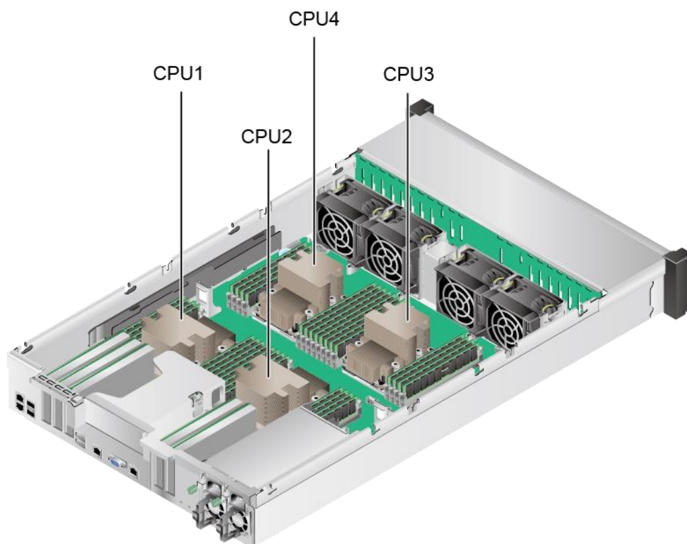
图5-13 处理器位置
