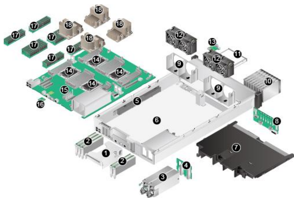
图3-1 2488 V5 物理结构（示例：8x2.5 英寸硬盘配置）
