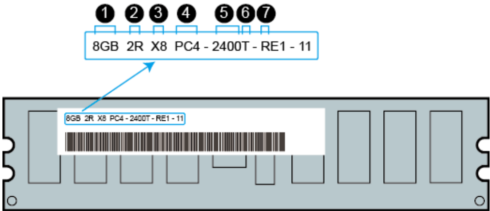
图5-14 内存标识
