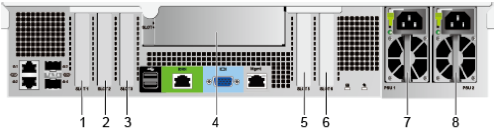
图5-10 后面板外观
