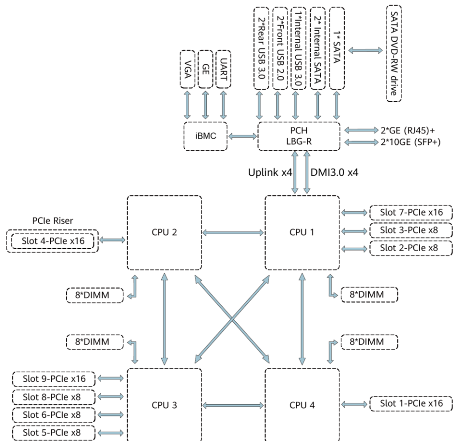
图4-1 2488 V5 逻辑结构
