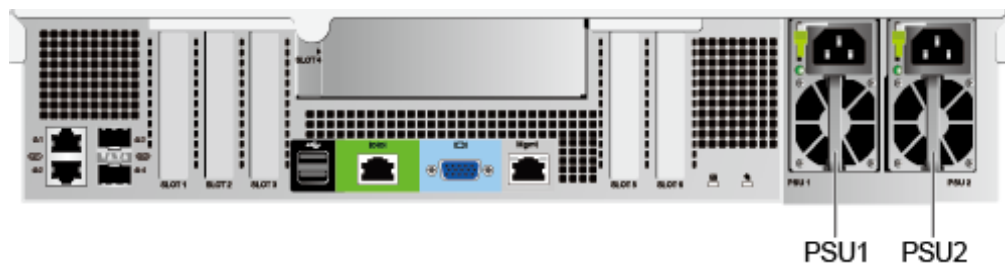
图5-26 电源位置
